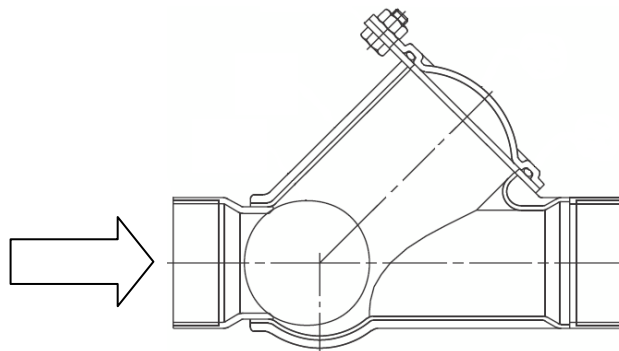
Montage Horizontal
